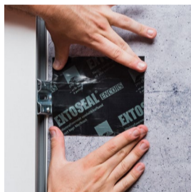
Wasserführende Verklebung von Befestigungswinkeln.
