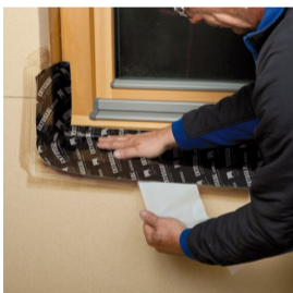
Einsatz als wasserdichte Unterfensterbank.
